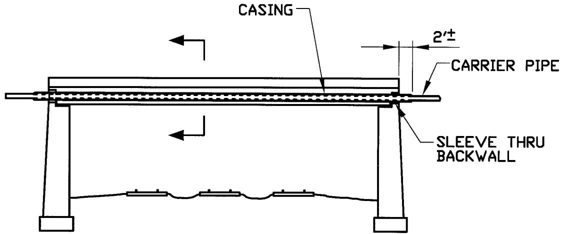
ELEVATION
